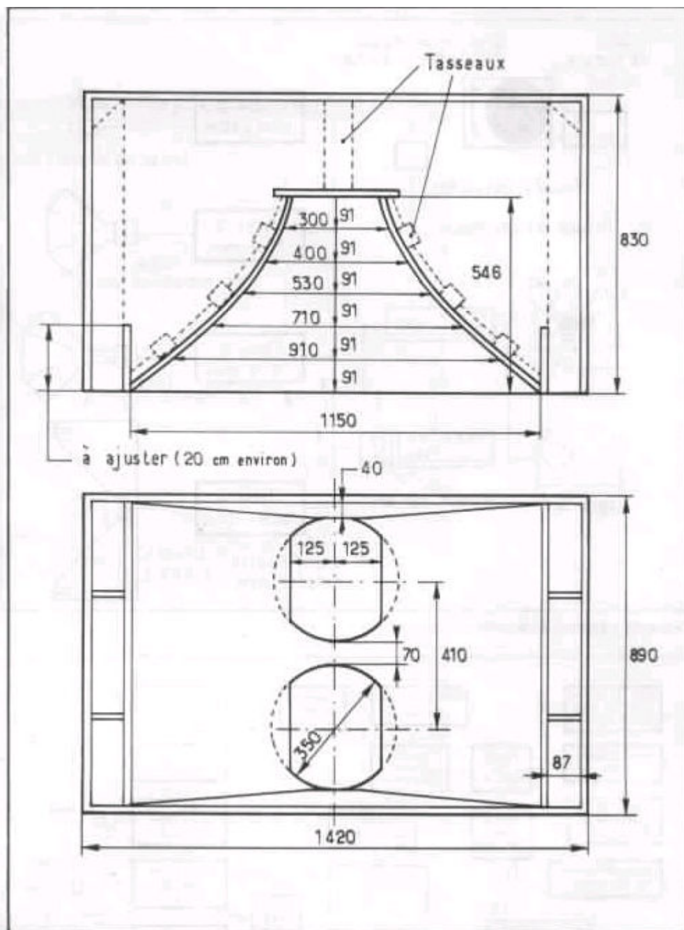
Fig 4 : Encelinte Onken, seconde version, à pavillon frontal, utilisant deux haut-parleurs Altec 515B.
